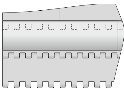
Standardanordnung S6.1-0 FLT PSU-16
