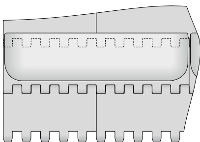
Standardanordnung S6.1-0 FLT BPU
