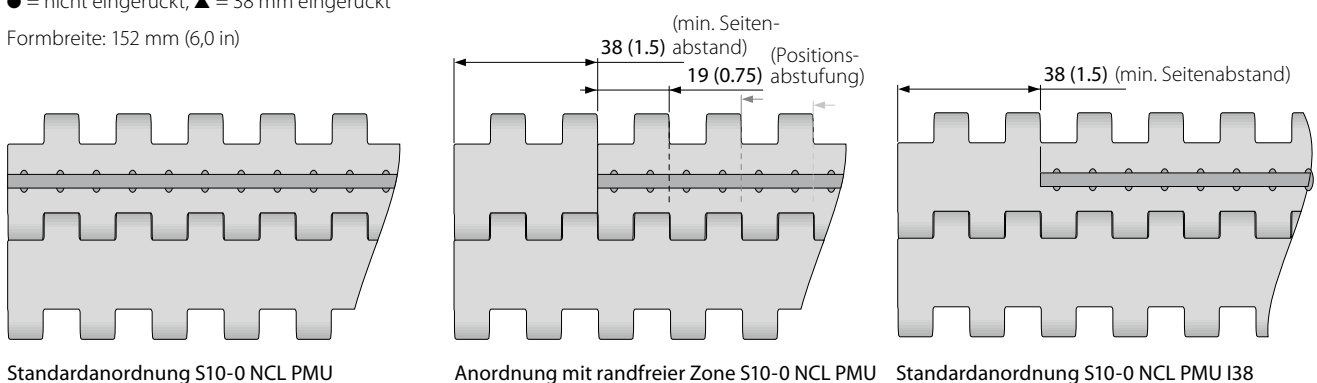
Standardanordnung S10-0 NCL PMU
