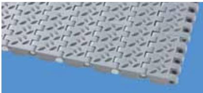
S8 | geschlossene Oberfläche | rutschfest (Design 2)
