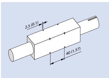
Welle 40 x 40 mm. Befestigen des Zahnrads mithilfe von Sicherungsringen gemäß DIN 471 (Seegerring), d = 56 mm. Die genauen Abmessungen sind im Anhang aufgeführt: Seite VI-11 .
