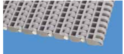
S8 | durchlässige (25%) Oberfläche | abgerundete Auflagefläche
